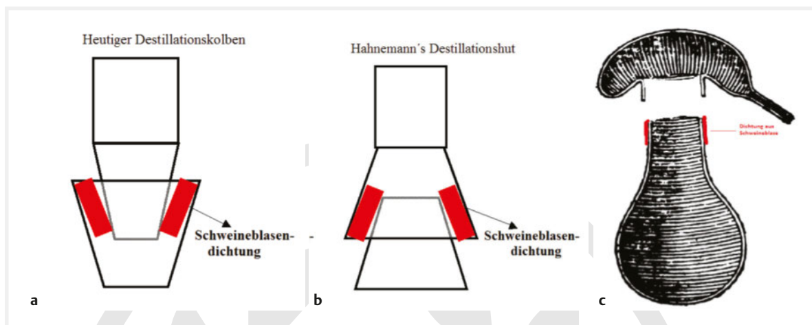
► Abb. 3 Destillationshelme und Anbringung der Schweineblasendichtung. Zeichnung der Destille aus dem Apothekerlexikon von Hahnemann.
