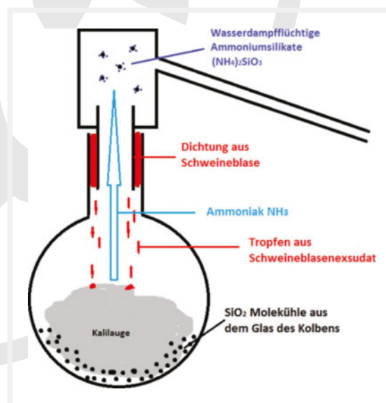
► Abb. 4 Entstehung von Ammoniak aus der Dichtung und von hydratisierten Silikaten aus dem Glaskolben in Verbindung mit heißer Kalilauge. In der Gasphase bilden sich schließlich Ammoniumsilikate.
