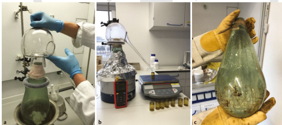
► Abb. 2 Destillationsverfahren mit Schweineblase als Dichtung; a Aufkleben des Helmes mit nasser Blase auf originalen Kolben und Alambik aus der Zeit ca. 1800–1840 [11]; b Original-Versuchsaufbau; c Kolben nach Causticum -Destillation mit Sprung. Bild a aus HK 1/2018 „Die Entschlüsselung des Causticumsrätsels“, mit freundlicher Genehmigung der Mediengruppe Oberfranken.
