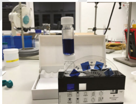
► Abb. 5 Photometrischer Nachweis von Silikaten im Destillat.
