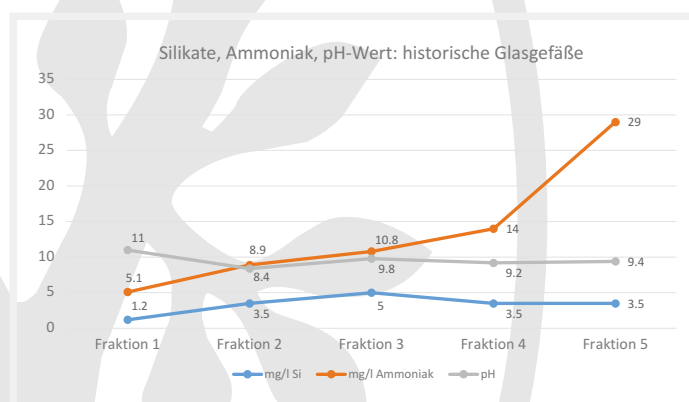
►Abb. 7 Fraktionierte Abnahme F1–F5, Entwicklung von Silikat, Ammoniak und pH-Wert.
