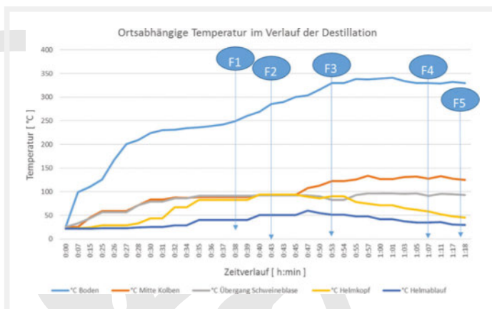
►Abb. 6 Temperaturentwicklung an verschiedenen Stellen des Destillationsaufbaus, Abnahmepunkte der Einzelfractionen F1 – F5.
