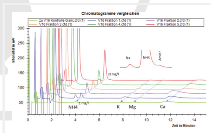
►Abb. 8 Kationenprofile der einzelnen Fraktionen (F1 – F5 und Reinwasserdestillation) der Destillationsversuche mit Originalgefäßen und Schweineblasendichtung (V16) in der HPLC-Analyse.
